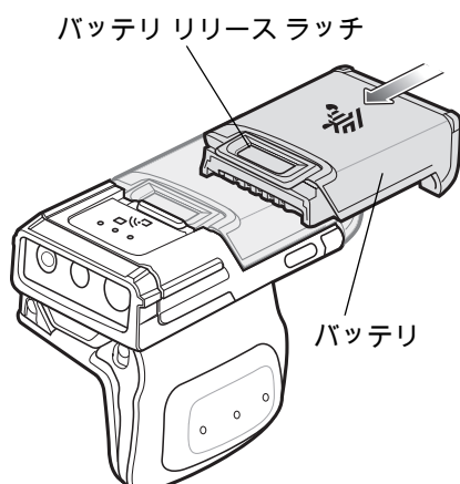
図2 バッテリーの取り付け
