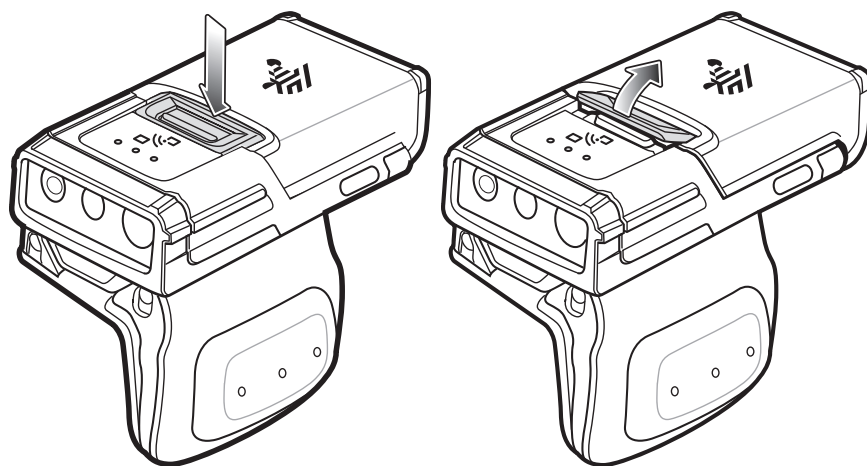
図3 バッテリーの取り外し
