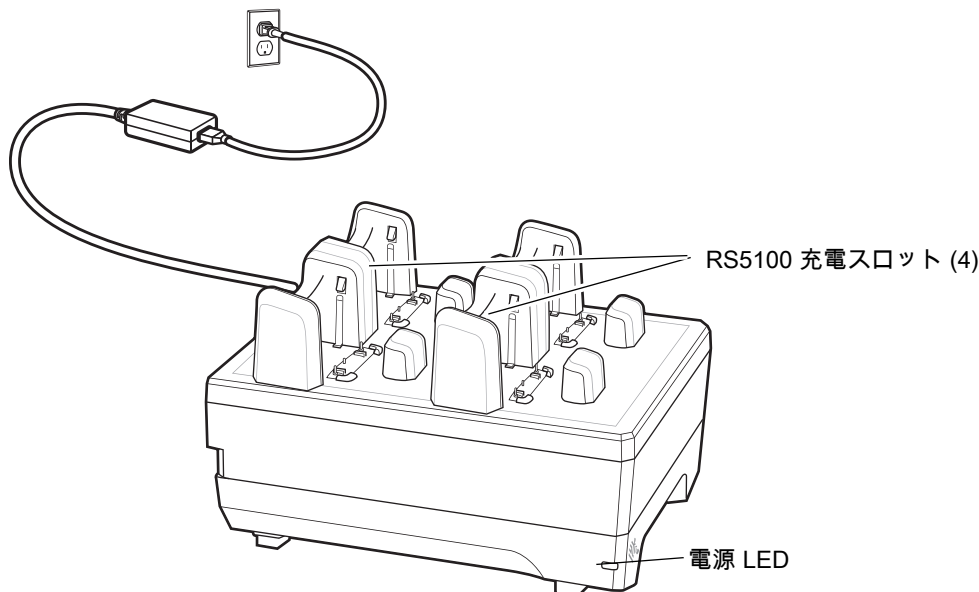
図 9 4 スロット RS5100 充電専用クレードル
