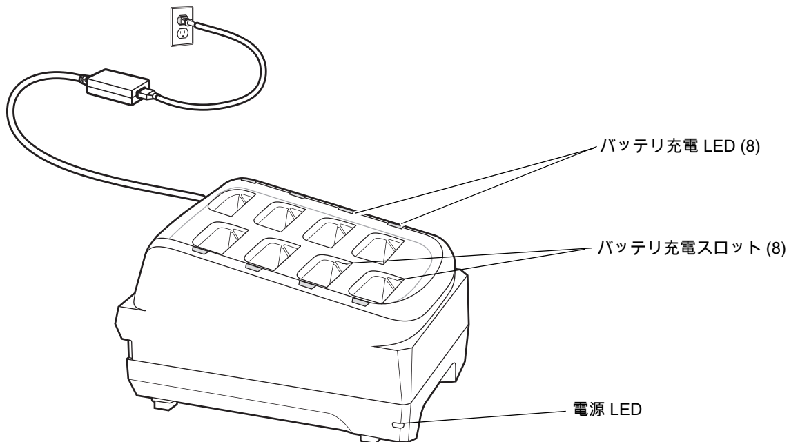
図 10 8 スロット バッテリー充電器
