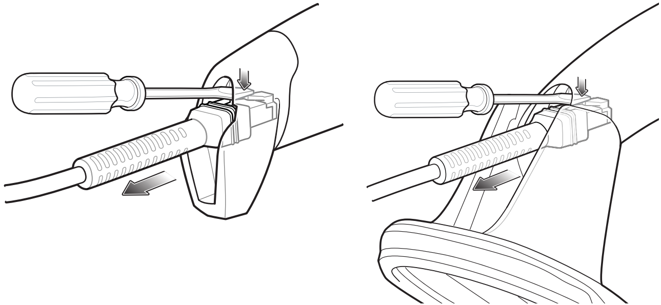
図 1-3 ケーブルの取り外し - DS4308 および DS4308P
