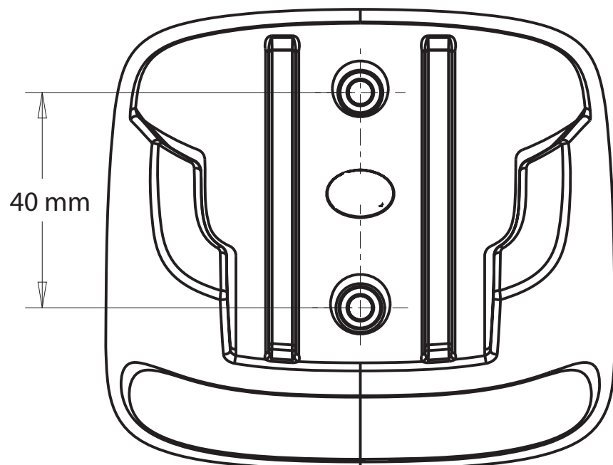
図 1-8 垂直設置ブラケットのテンプレート
